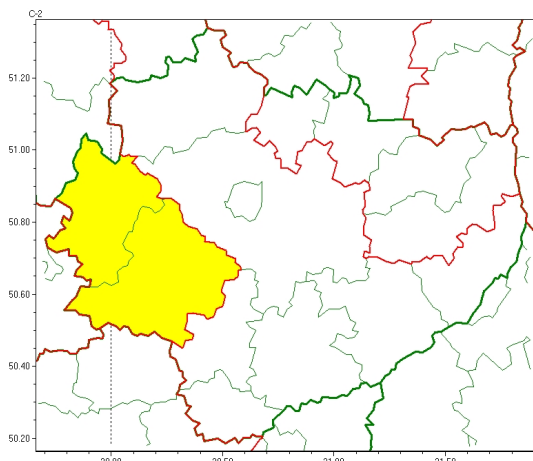
Opady marznące 2026-01-13 18:50
