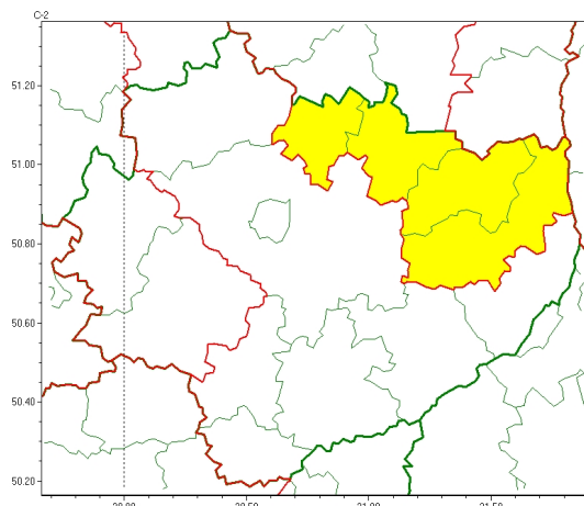
Silny mróz 2026-01-13 18:50
